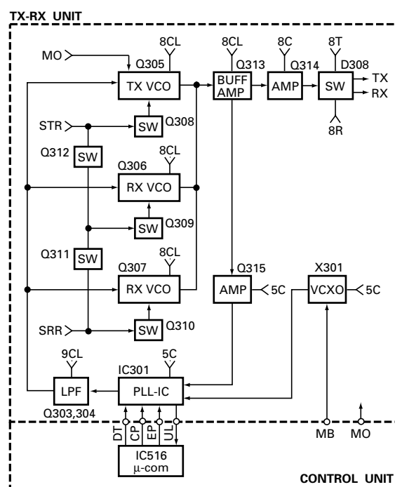
Fig. 9 VCO/PLL circuit
