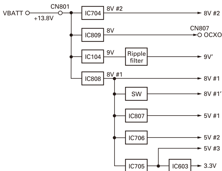
Fig. 8 AVR circuit
