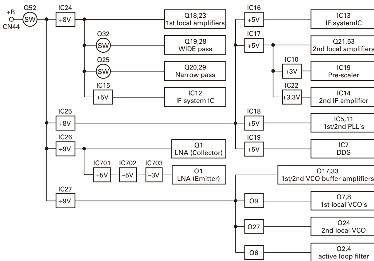
Fig. 22 AVR circuit
