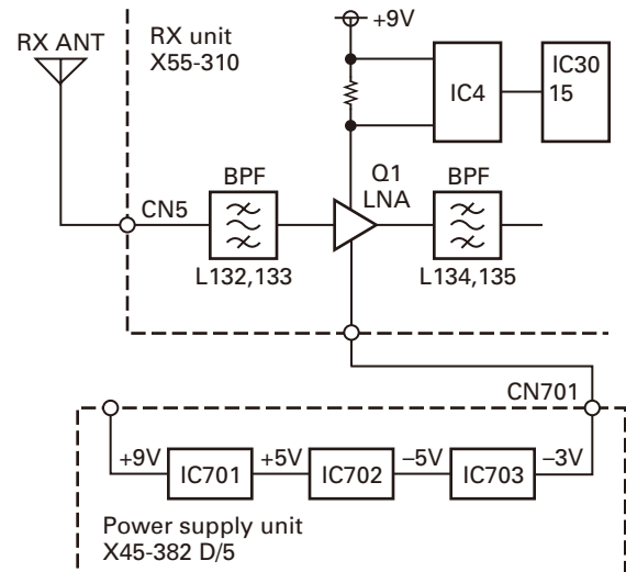
Fig. 16 Front-end circuit
